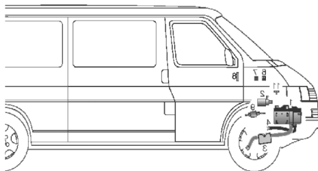
Рис.3. Отопительный прибор в грузопассажирском автомобиле
