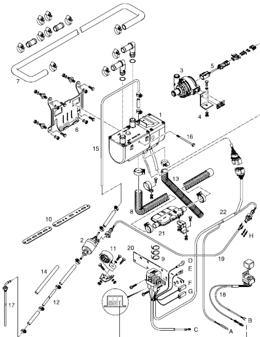
Рис. 5. Комплект поставки отопительного прибора, работающего на бензиновом/дизельном топливе
