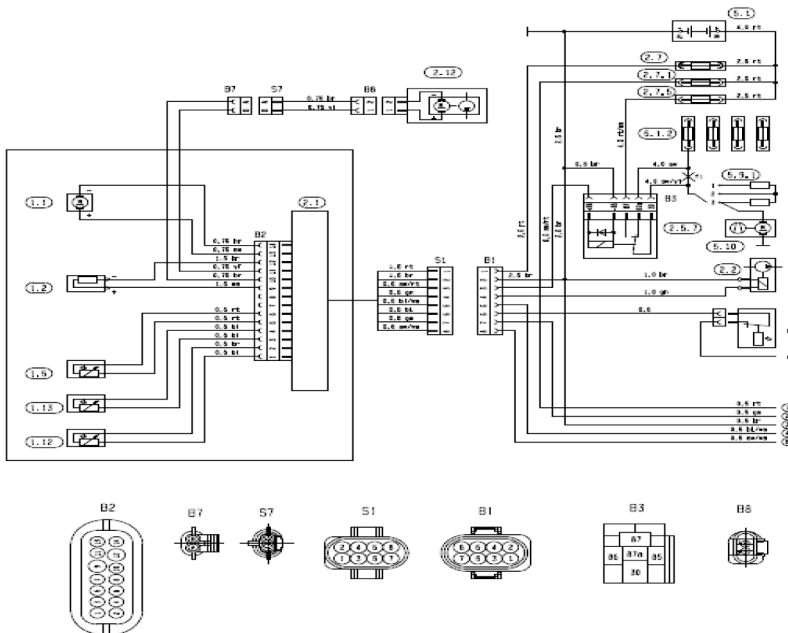
Рис. 6. Схема электрооборудования отопительного прибора
